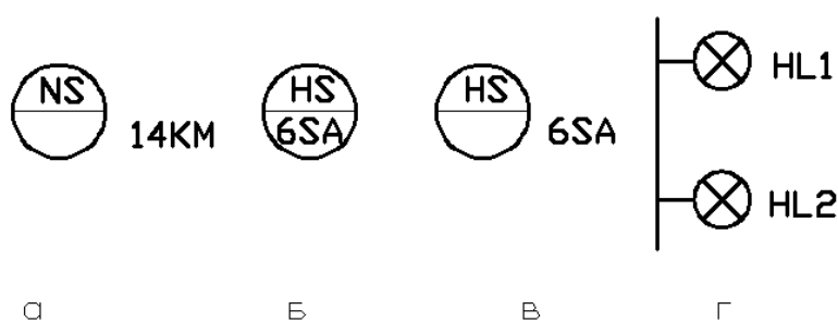
Рисунок 5.13 – Нанесение позиционного обозначения прибора на ФС по ГОСТ электрических принципиальных схем: а – переключатель цепей управления в 14-ом контуре, магнитный пускатель; б, в – переключатель кнопочный в 6-ом контуре; г – сигнальные лампы
