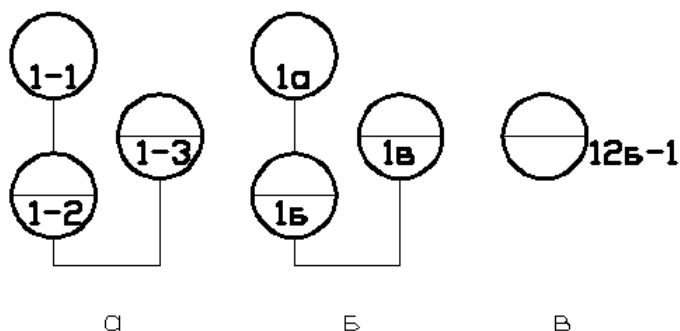
Рисунок 5.12 – Пример нанесения позиционного обозначения прибора: а – цифровой код; б – цифро-буквенный код; в – нанесение позиционного обозначения рядом с условным графическим обозначением
