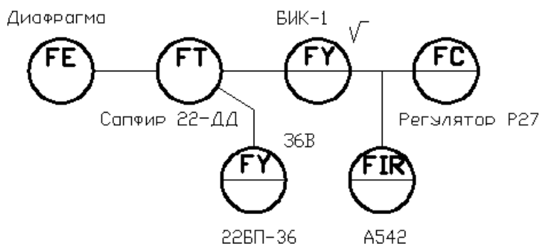
Рисунок 5.8 – Пример обозначения приборов, входящих в контур регулирования
