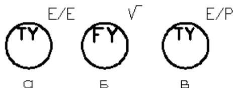
Рисунок 5.7 – Нанесение надписей вида преобразования рядом с графическим обозначением прибора: а – измерительный преобразователь, преобразующий сигнал термопары в унифицированный электрический сигнал постоянного тока; б – блок извлечения корня БИК-1; в – преобразователь электрического сигнала в пневматический
