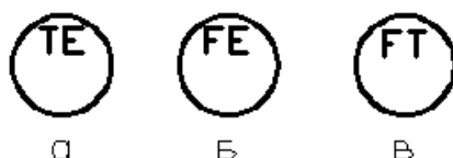
Рисунок 5.6 – Построение условного обозначения приборов с использованием дополнительных буквенных обозначений функциональных признаков приборов: а – термопара, термометр сопротивления; б – диафрагма; в – «Сапфир-22-ДД».
